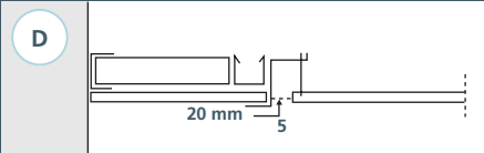
Frisprofil, fast fris
