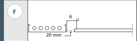
Fast Fris monterat med kabelrännaprofil
